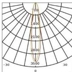
Curva 11,7W
