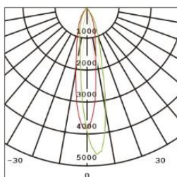
Curva 15,8W
